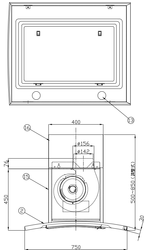
底面図
