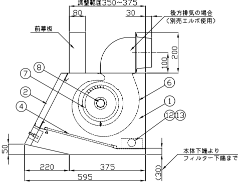
背面取付図
