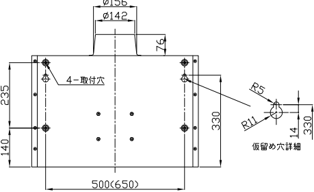
背面取付図
