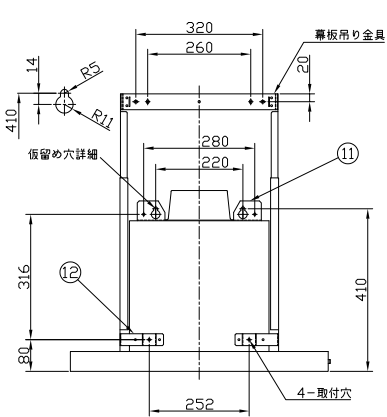
背面取付図
