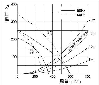
□静圧 - 風量曲線
