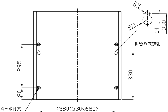
背面取付図
