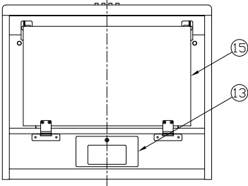
底面図
