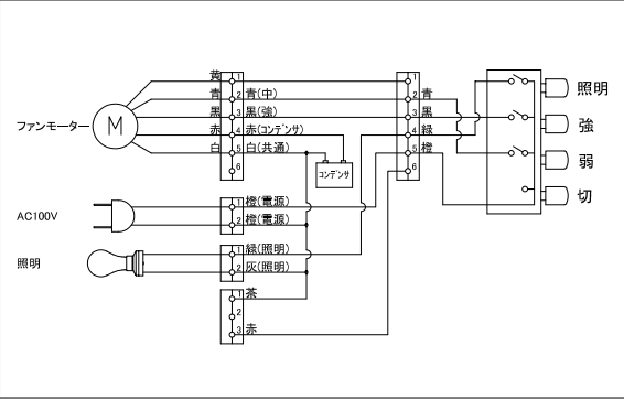
□結線図
