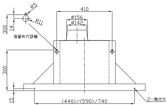
背面取付図
