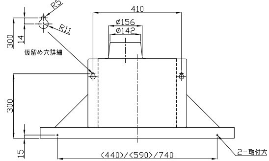
背面取付図
