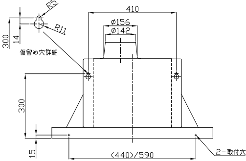
背面取付図
