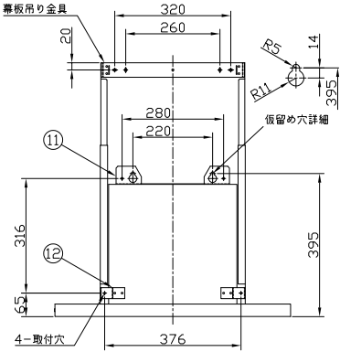
背面取付図
