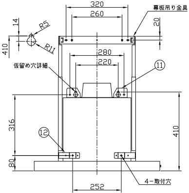
背面取付図
