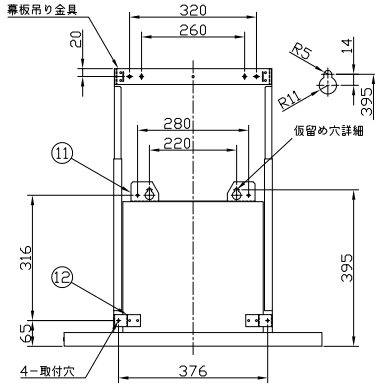
背面取付図
