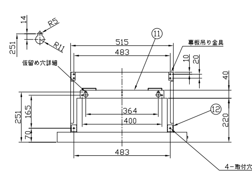
背面取付図
