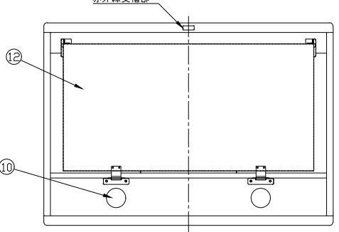
底面図
