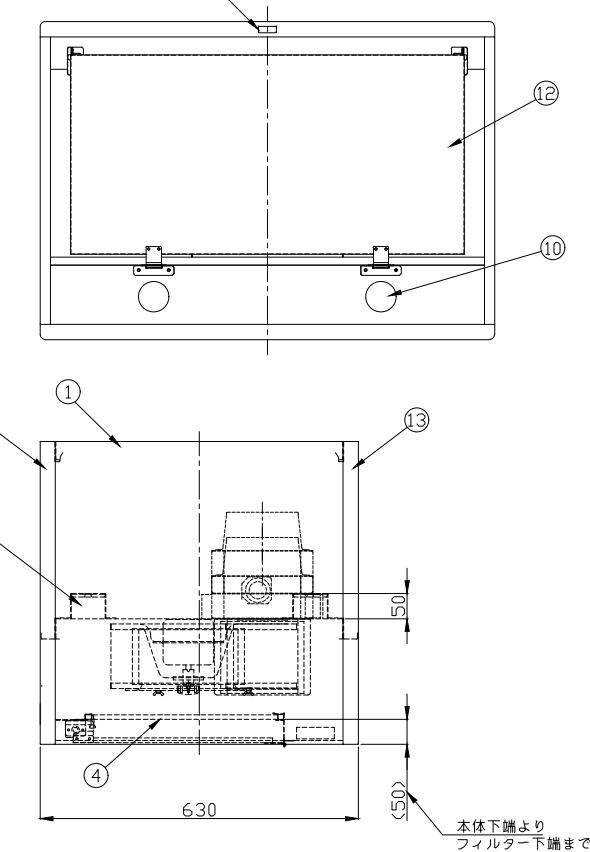
底面図
