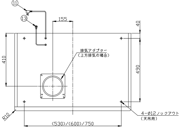
底面図
