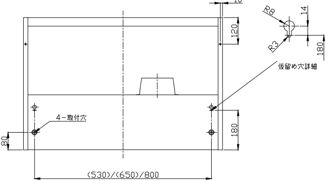
背面取付図
