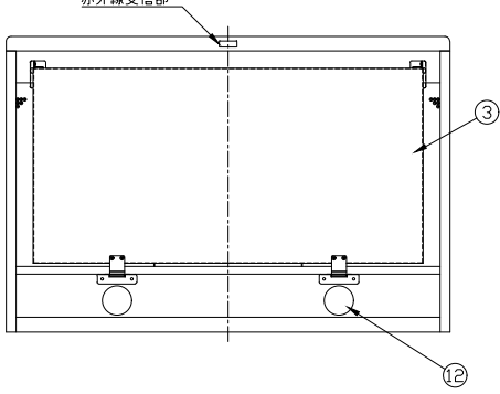
後方排気の場合 (別売エルボ使用)
