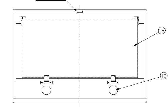
底面図
