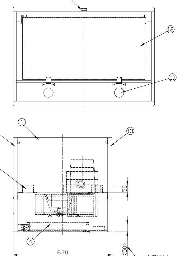
底面図
