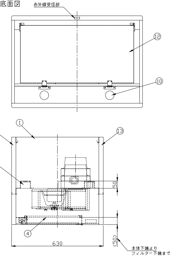
底面図
