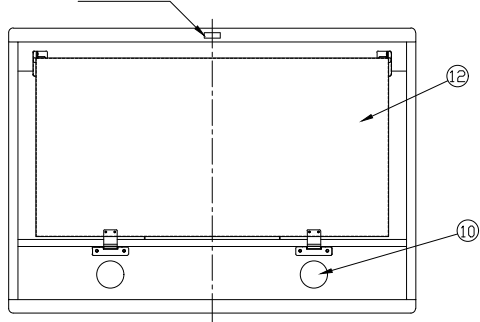
底面図 赤外線受信部
