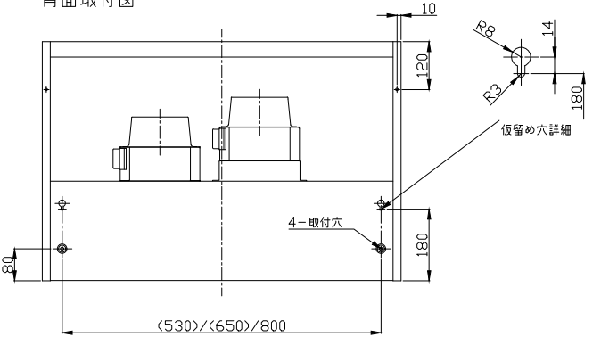
背面取付図
