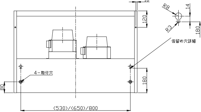
背面取付図
