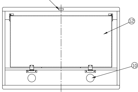
底面図
