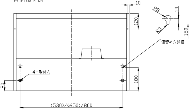
背面取付図
