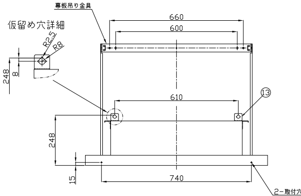
背面取付図
