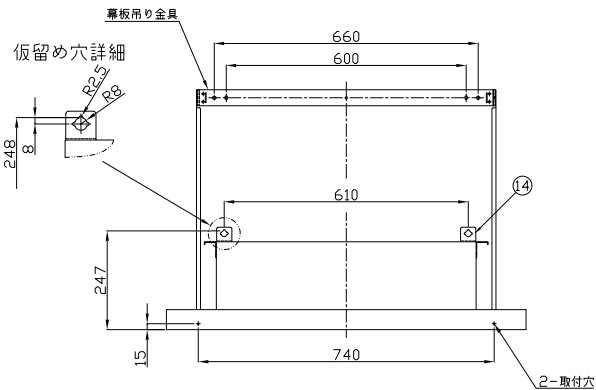
背面取付図
