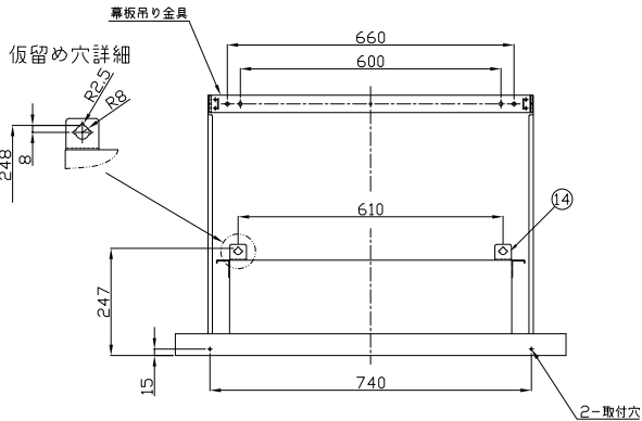
背面取付図
