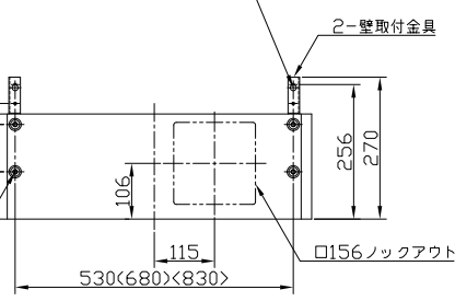
背面取付図
