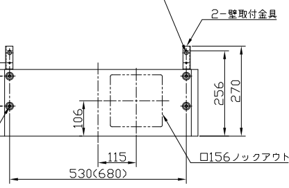
背面取付図
