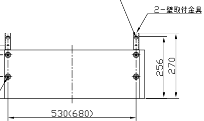
背面取付図
