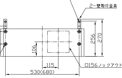
背面取付図
