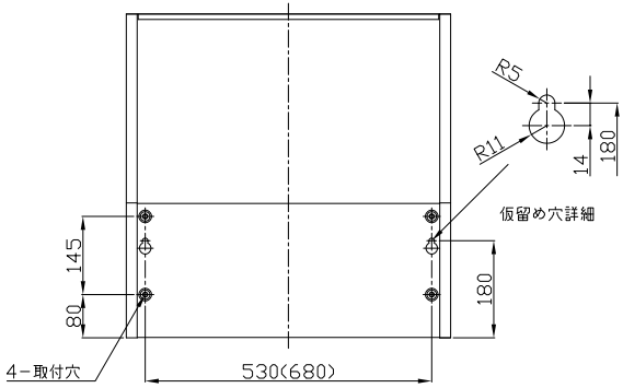
背面取付図
