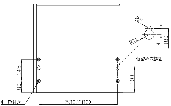
背面取付図
