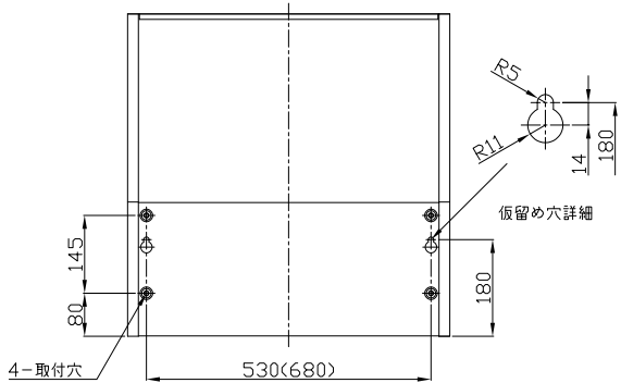
背面取付図
