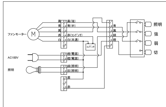
□結線図
