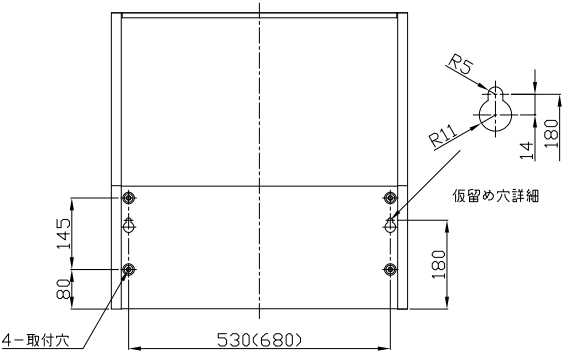
背面取付図
