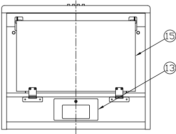
底面図
