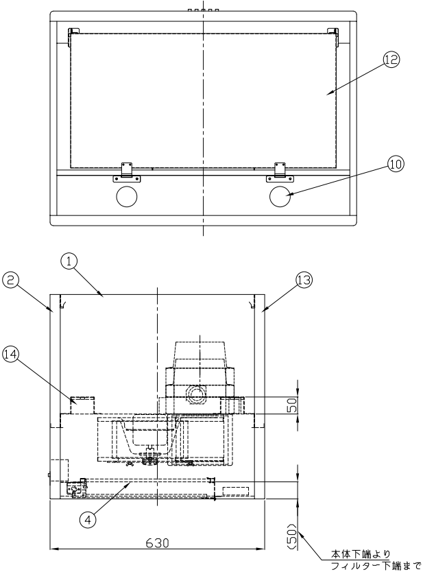
底面図
