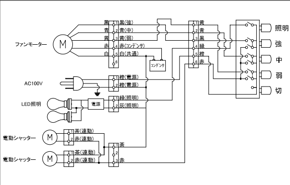
□ 結線図
