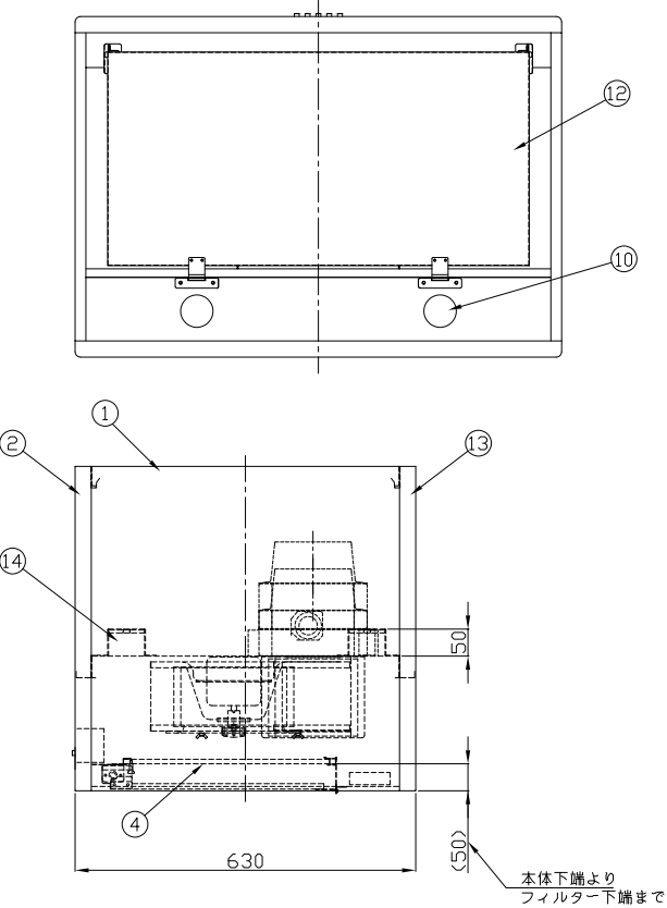
底面図
