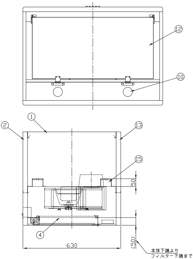
底面図
