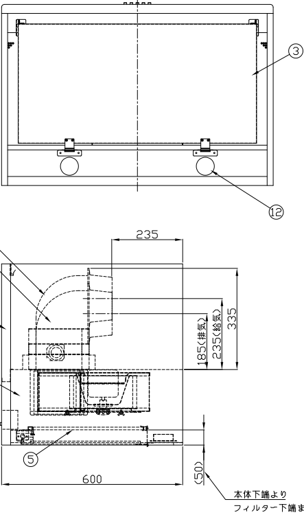
底面図
