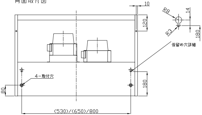
背面取付図
