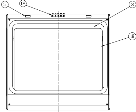
底面図
