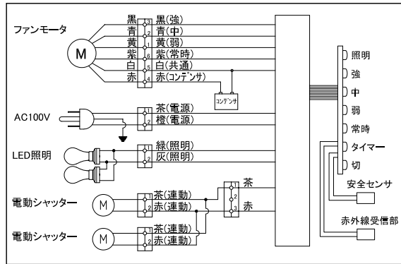
□結線図
