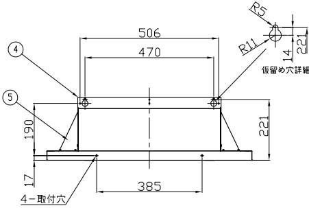
背面取付図
