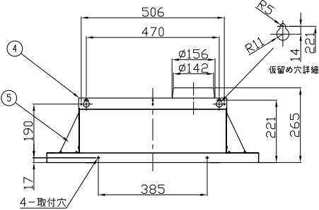
背面取付図
