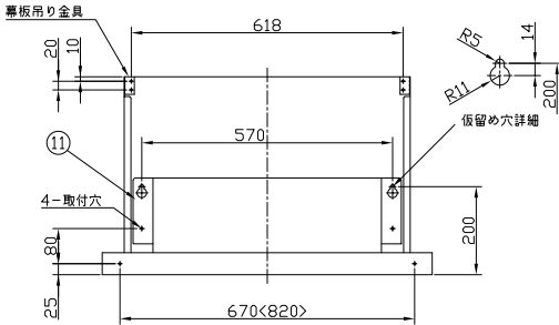
背面取付図
