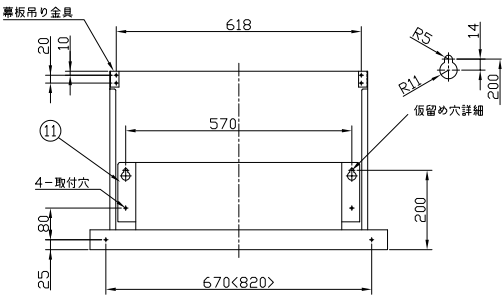
背面取付図
