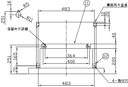
背面取付図
