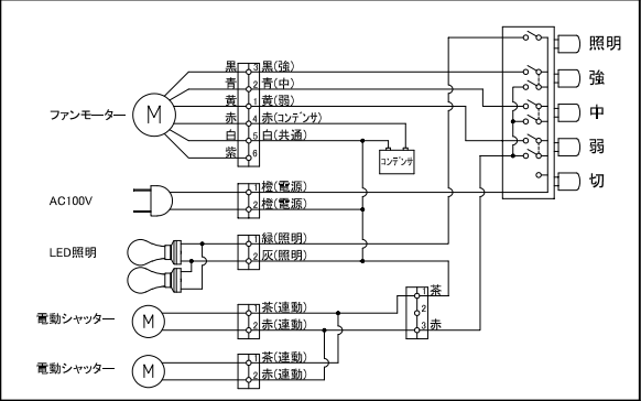
□ 結線図
