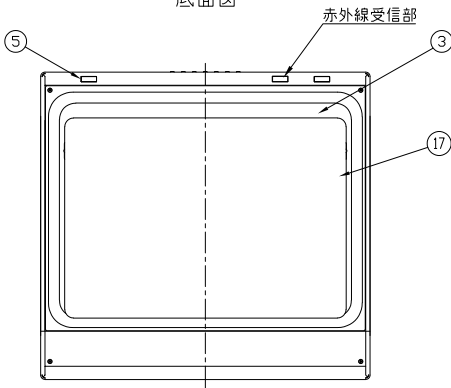
底面図
