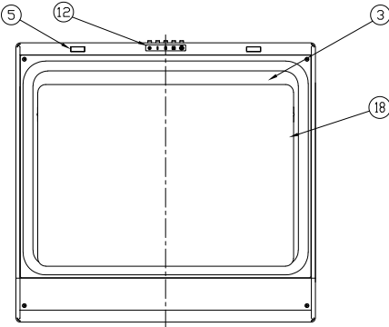
底面図
