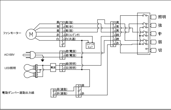
□結線図
