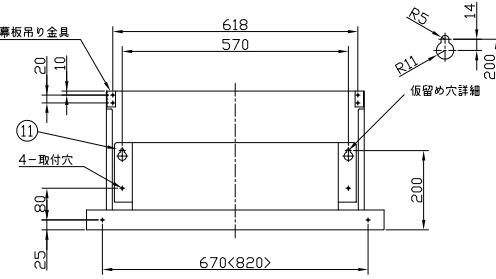
背面取付図
