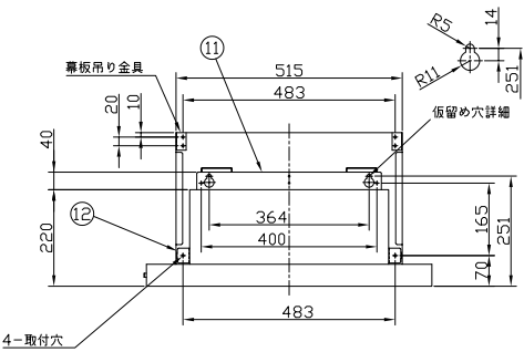
背面取付図
