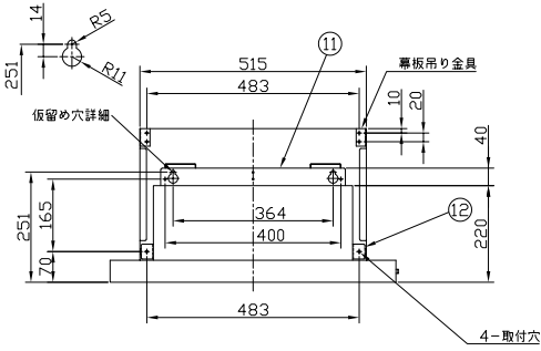
背面取付図
